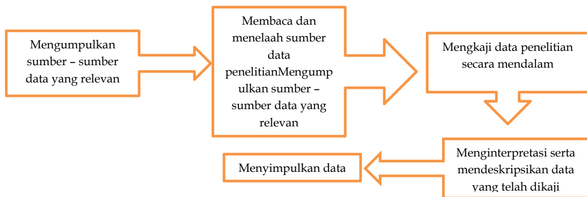
Gambar 1. Desain penelitian
